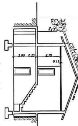
Sezione A-A
