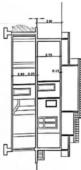
Sezione B-B
