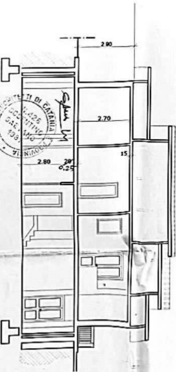
Sezione B-B
