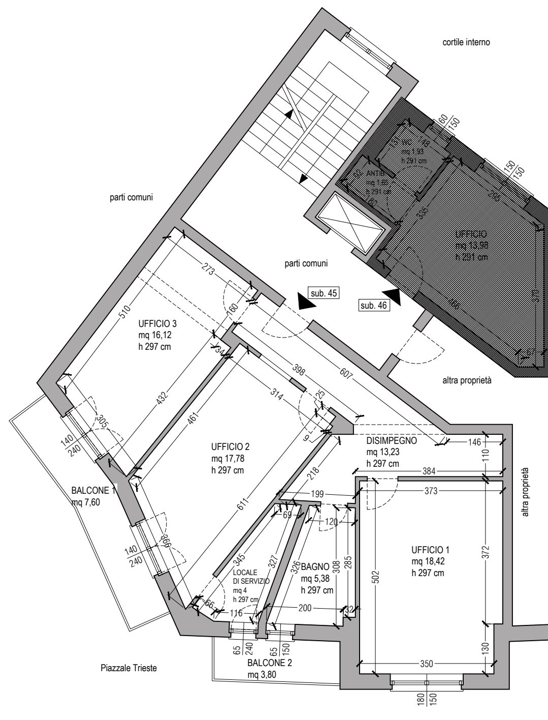
PIANTA STATO DI FATTO sub. 45 PIANO QUARTO UFFICIO
