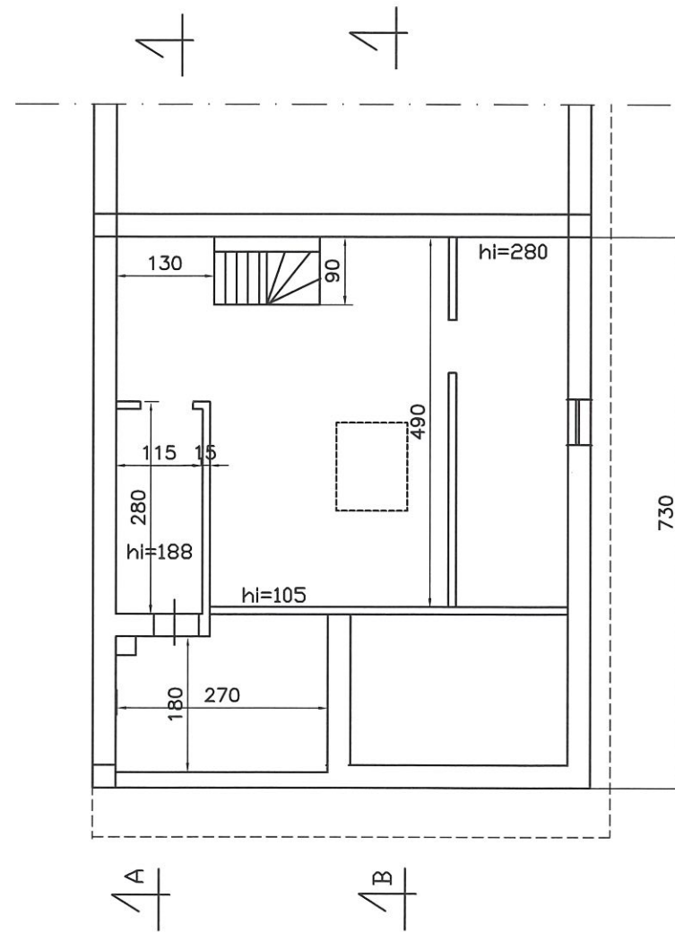
Piano sottotetto (Piano secondo)
