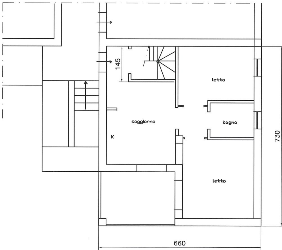
Piano primo
