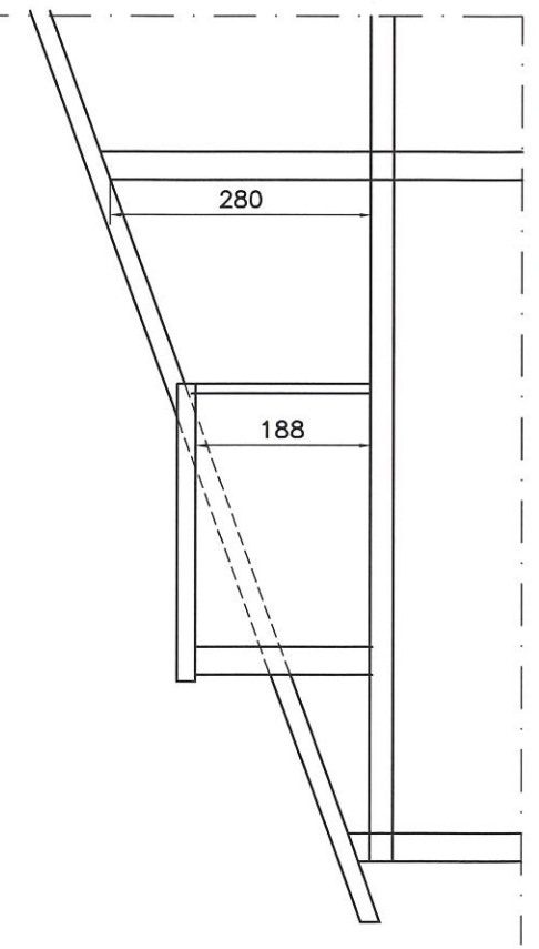
SEZ AA
