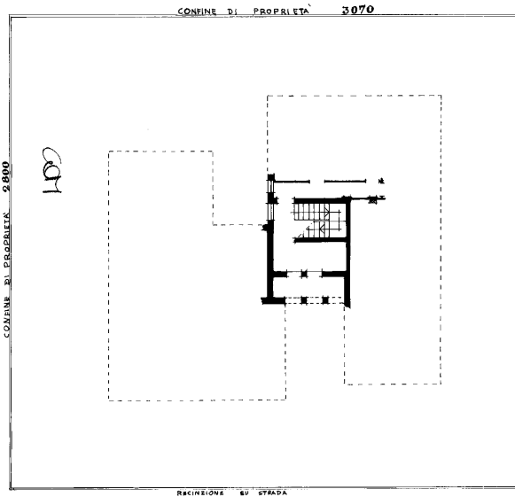
PIANTA PIANO TERRA - H 2.30
