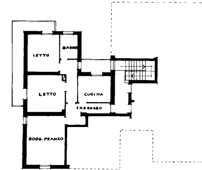
PIANTA PIANO SECONDO H 2.80
