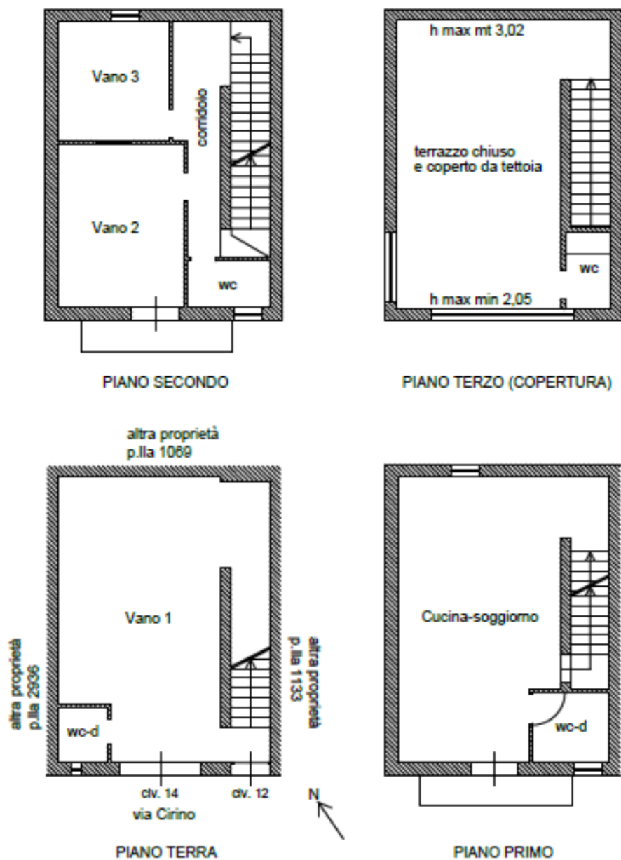
Planimetria dello stato reale dei luoghi in All. 12
