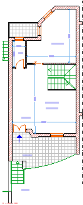
PIANTA PIANO TERRA scala 1/100
