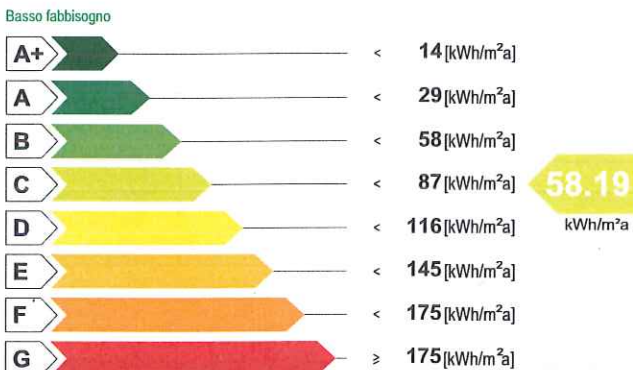
Fabbisogno termico per la climatizzazione estiva
