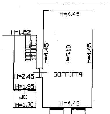
PIANO SECONDO
