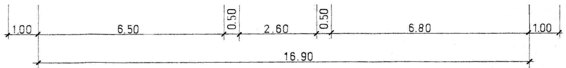
PIANTA LOCALE TECNICO E TERRAZZO CALPESTABILE
