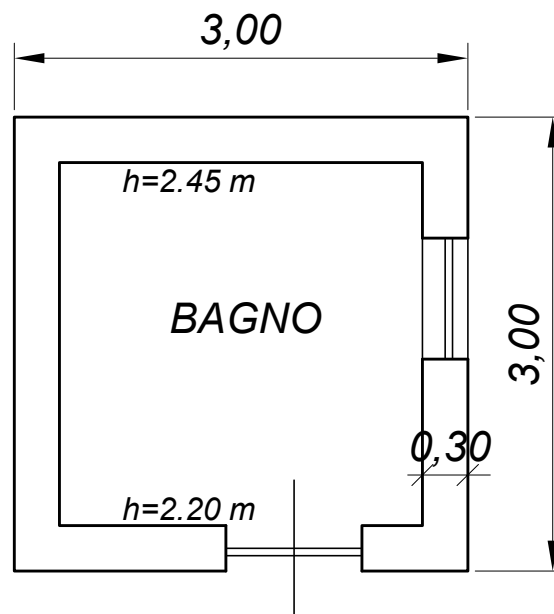
BAGNO PLANIMETRIA Rapp. 1:50
