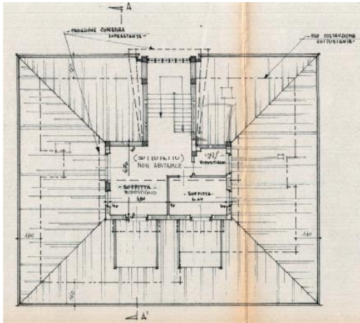
Estratto tavola grafica Lic. Ed. 49/1972 - piano sottotetto
