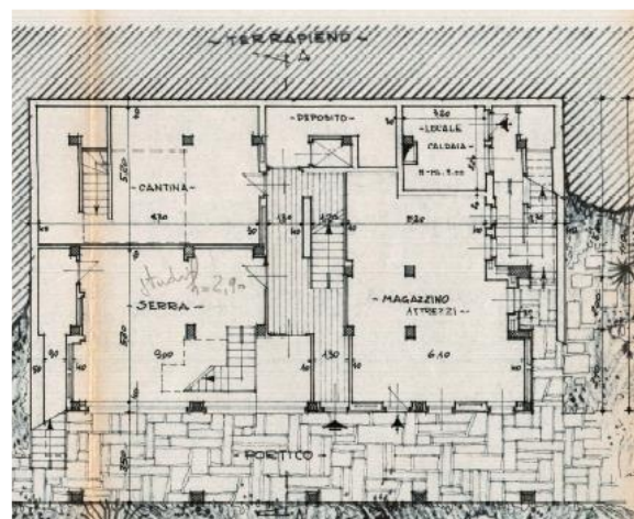
Estratto tavola grafica Lic. Ed. 49/1972 - piano seminterrato
