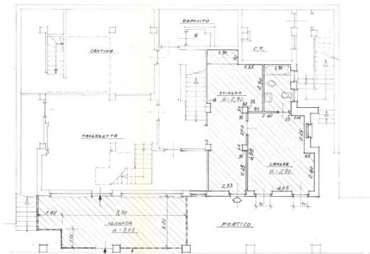
Estratto tavola grafica Concessione in sanatoria
