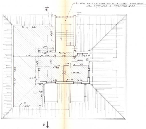
Estratto tavola grafica Concessione in sanatoria
