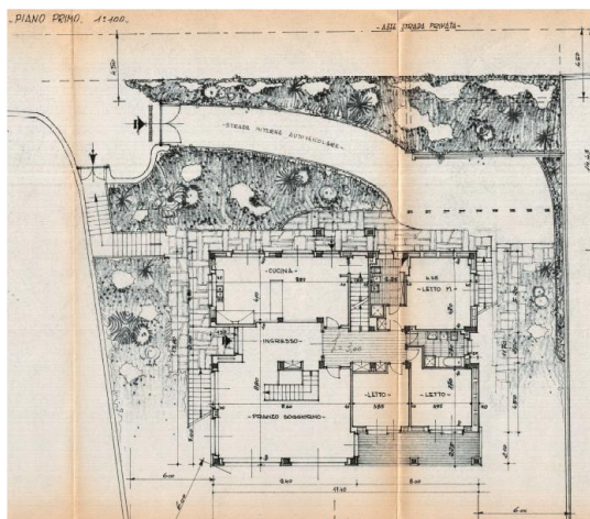
Estratto tavola grafica Lic. Ed. 49/1972 - piano 1°
