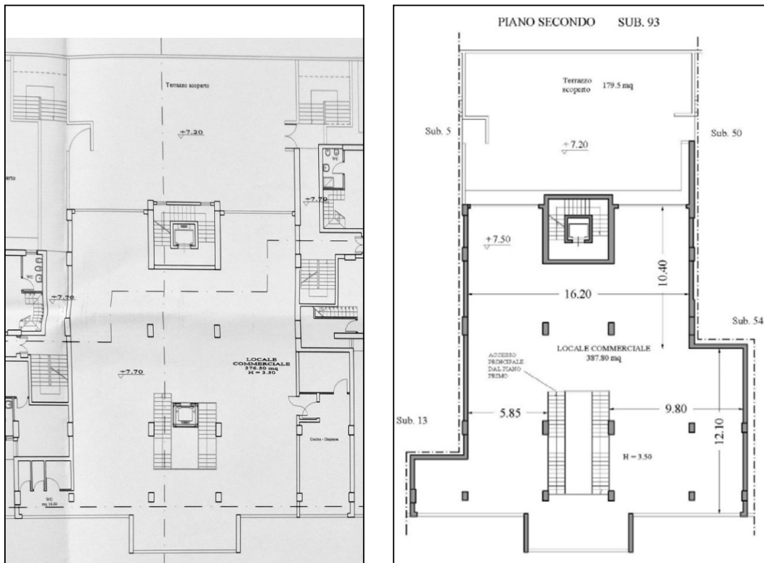
SECONDO PIANO - CONFORME
