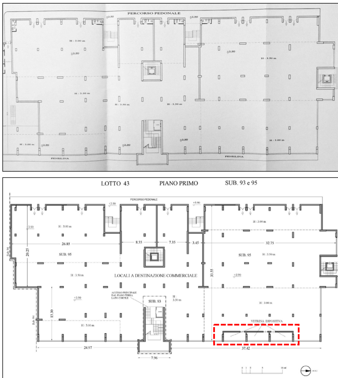
Fig. 5 – Confronto grafico SCIA con lo stato dei luoghi
