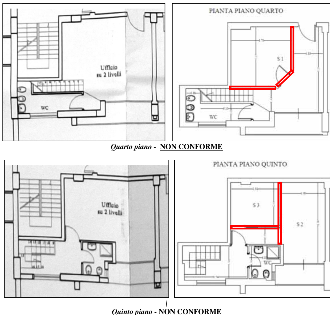
Fig. 6 – Confronto grafico PDC con lo stato dei luoghi – NON CONFORME
