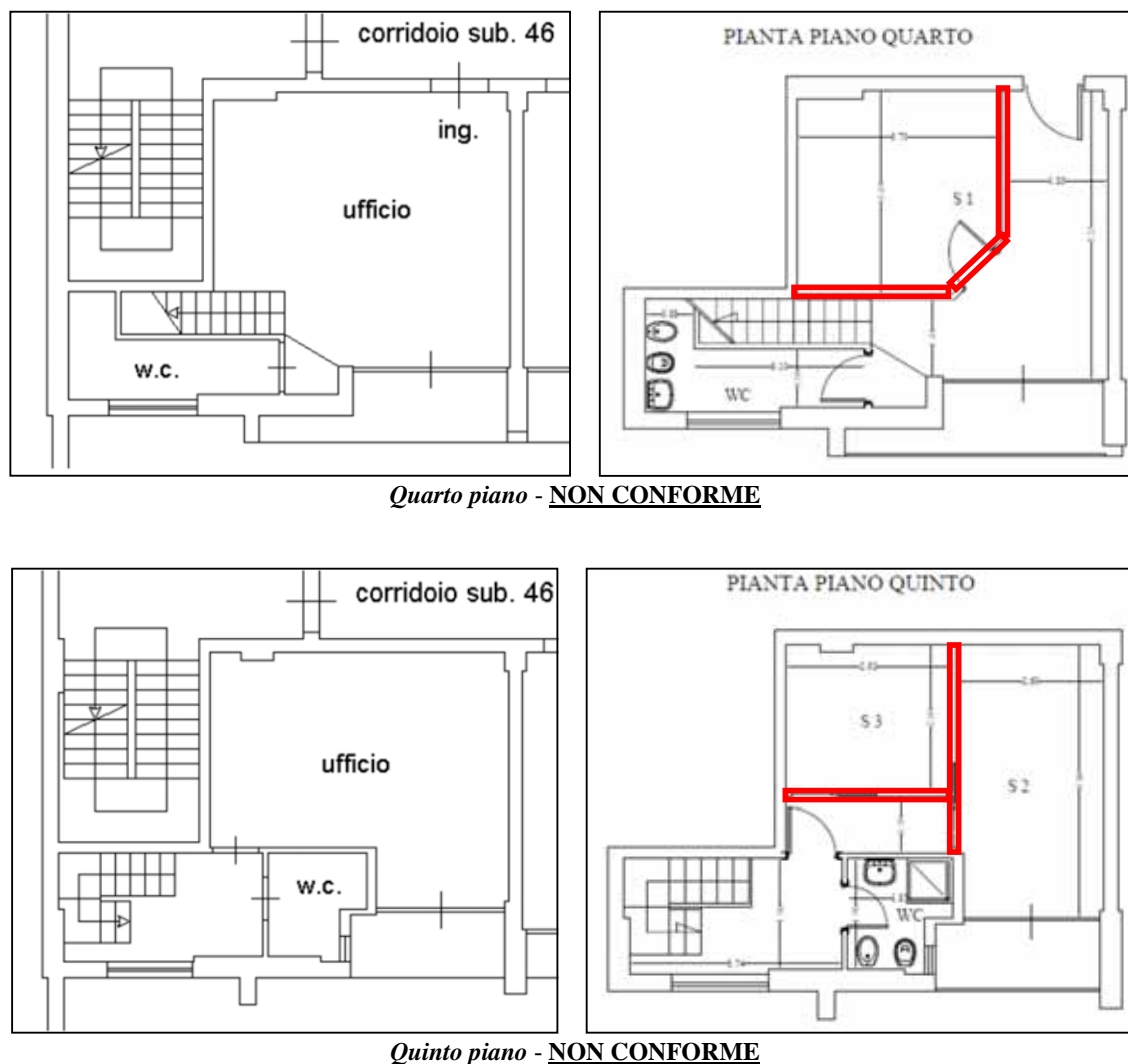
Fig. 5 – Confronto delle Planimetrie in atti al Catasto con lo stato dei luoghi - NON - CONFORME
