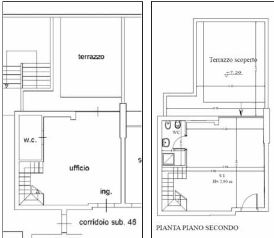
Fig. 5.1 - Confronto della Planimetria in atti al Catasto con lo stato dei luoghi 2° piano - CONFORME
