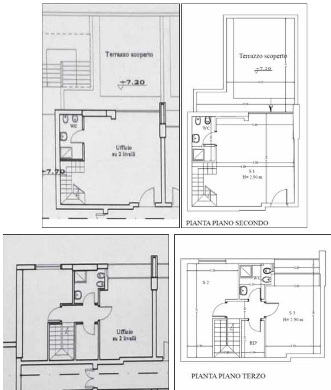
Fig. 6 - Confronto grafico PDC con lo stato dei luoghi - CONFORME
