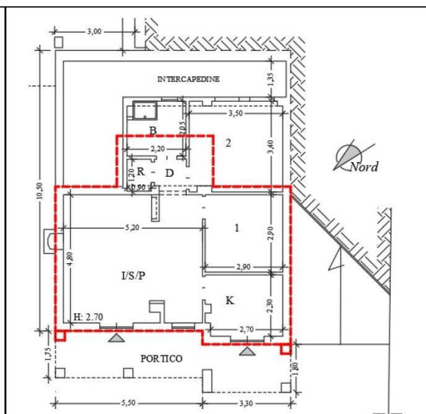
Figura 10 Pianta Piano Seminterrato - Stato di fatto con individuazione in rosso delle dimensioni dell'appartamento autorizzate con P.d.C. 16/2007
