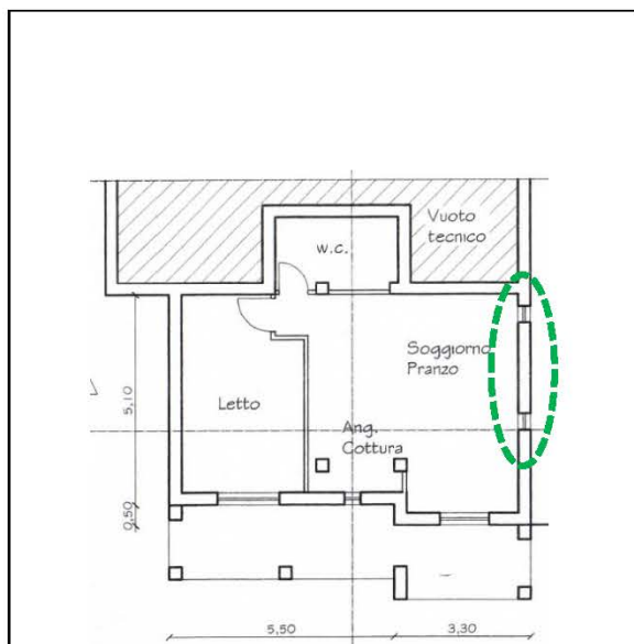
Figura 9 Pianta Piano Seminterrato allegata al P.d.C. 16/2007
