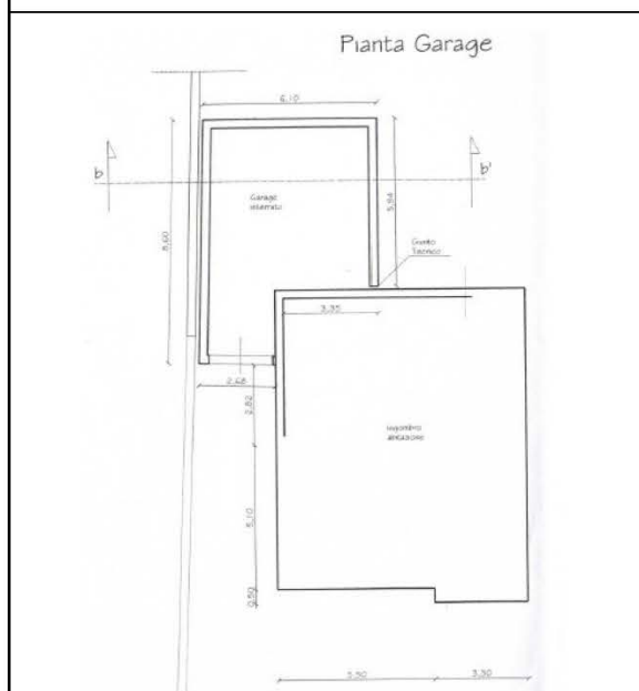
Figura 11 Pianta Piano Seminterrato allegata al P.d.C. 39/2008
