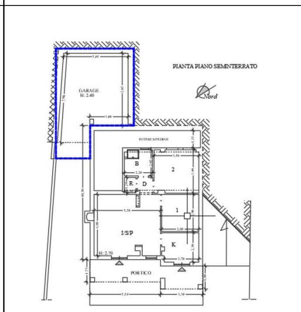
Figura 12 Pianta Piano Seminterrato - Stato di fatto con individuazione in blu delle dimensioni del garage autorizzate con P.d.C. 39/2008
