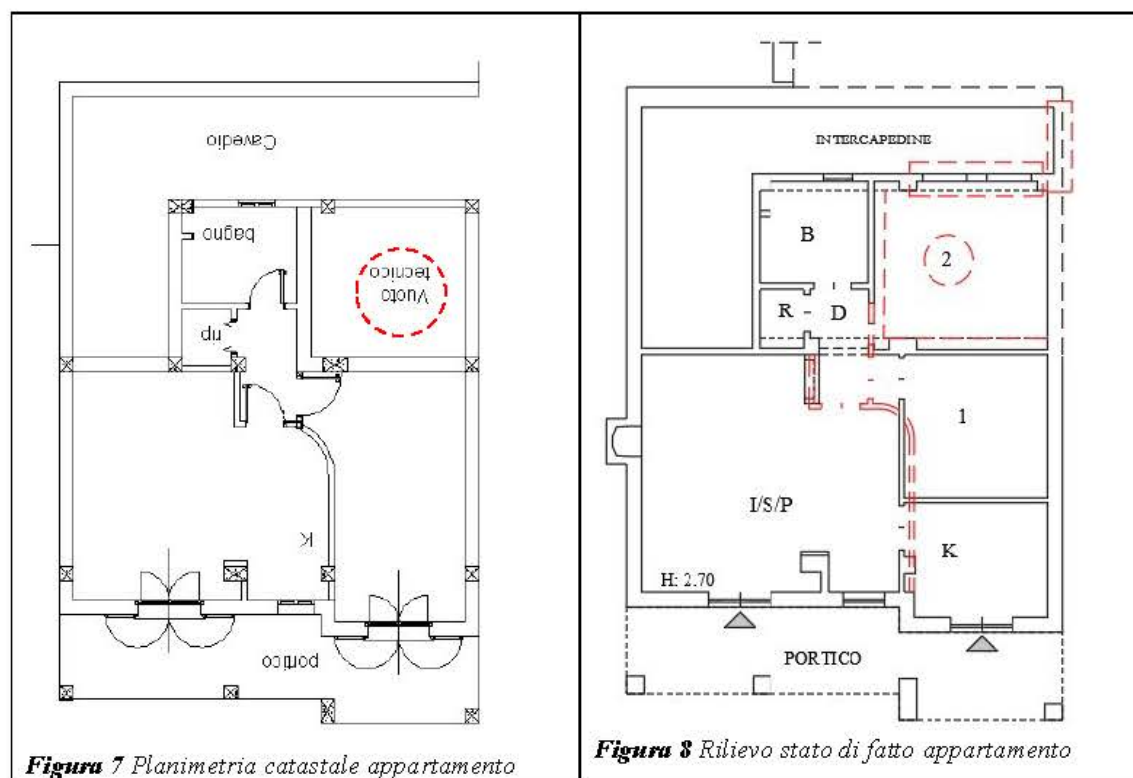
Figura 7 Planimetria catastale appartamento Figura 8 Rilievo stato di fatto appartamento Confronto tra planimetria catastale e pianta di rilievo dell'appartamento con individuazione in rosso delle difformità catastali riscontrate.
