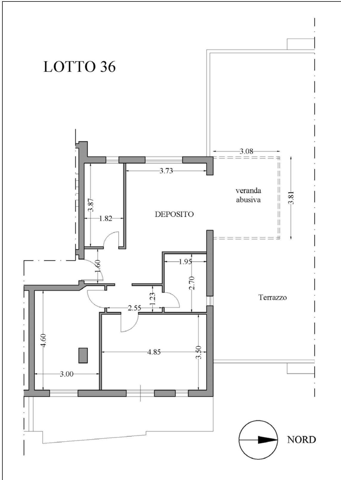
Fig. 3 - Pianta del rilievo dello stato dei luoghi
