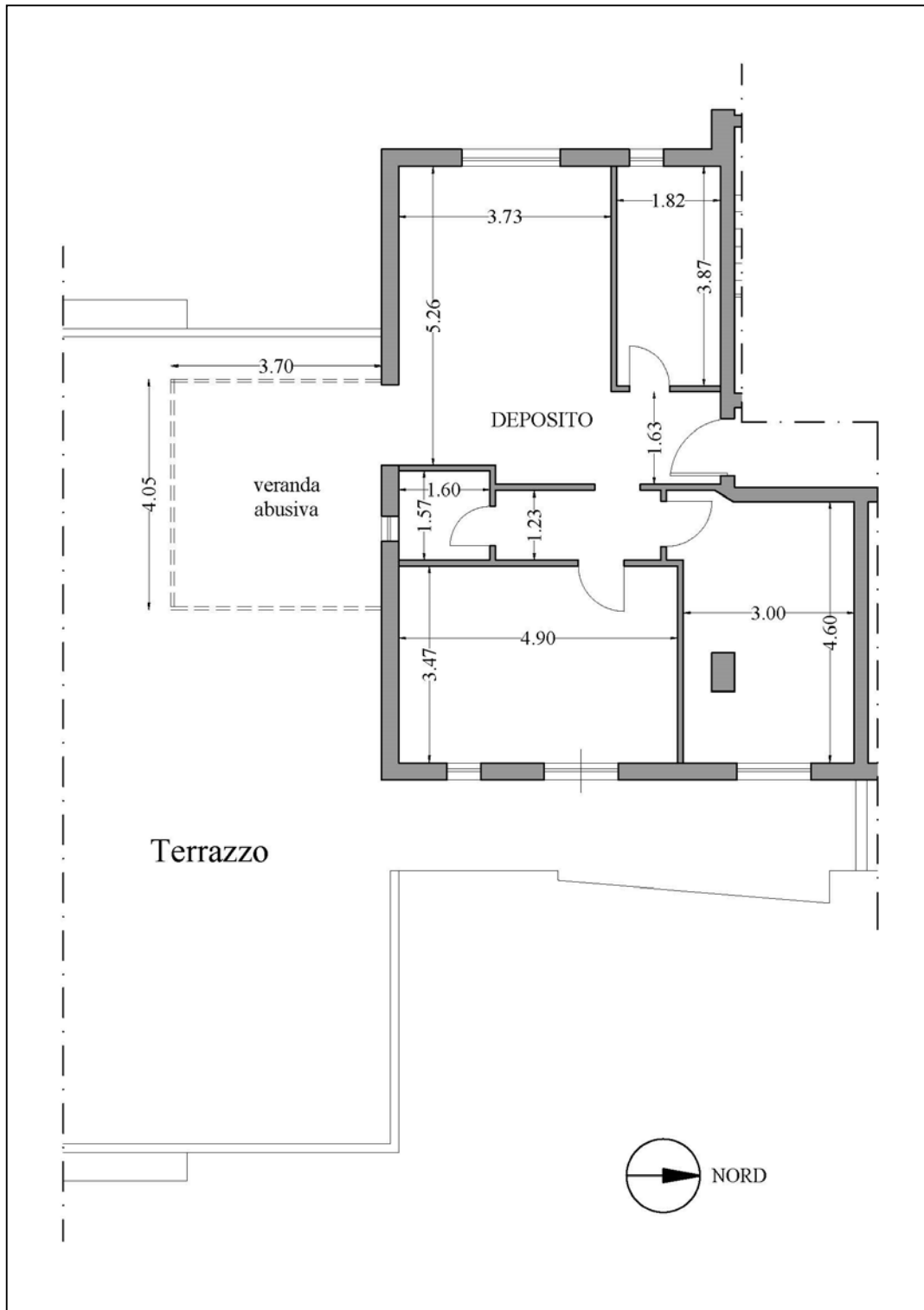
Fig. 3 - Pianta del rilievo dello stato dei luoghi
