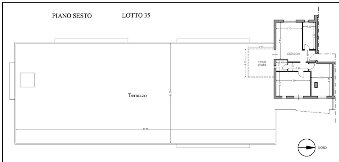
Fig. 2 - Pianta generale dello stato dei luoghi
