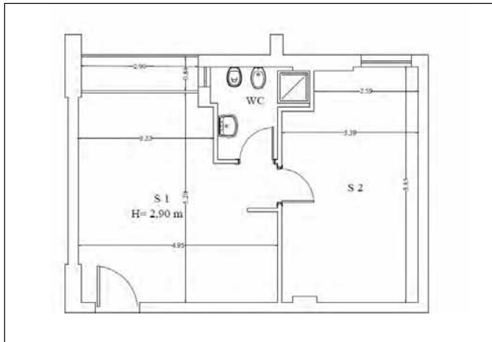
Fig. 2 – Pianta dello stato dei luoghi
