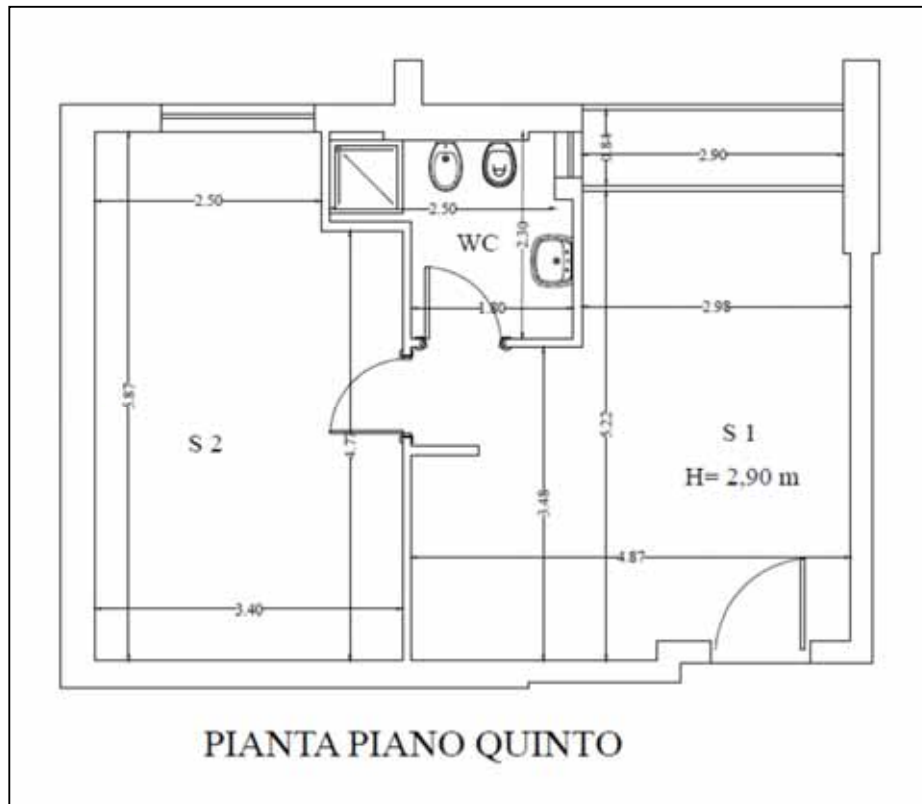
Fig. 2 – Pianta dello stato dei luoghi
