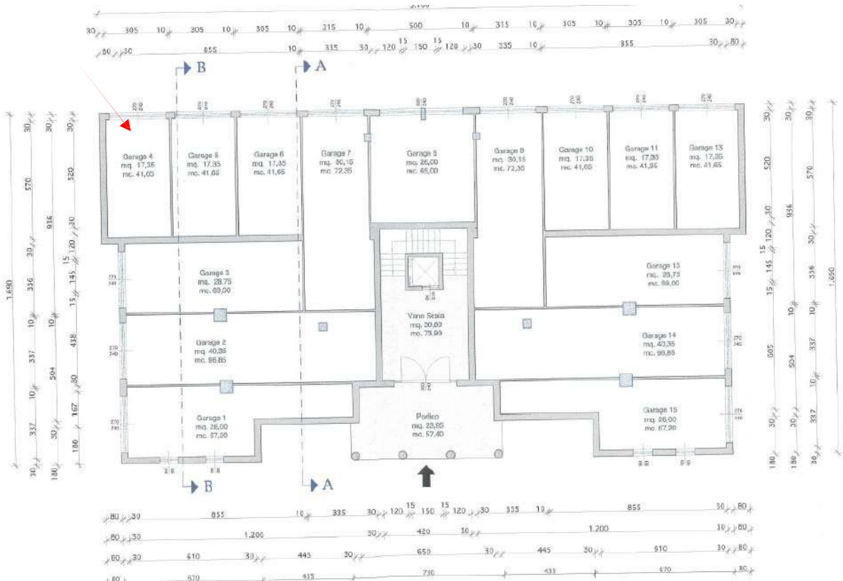
Figura 33. Stato approvato. (D.I.A. nr. 114.2/04 del data 29 aprile 2004) Autorimessa piano terra – fg.7 part. 1168 sub. 1 – GARAGE NUMERO 4
