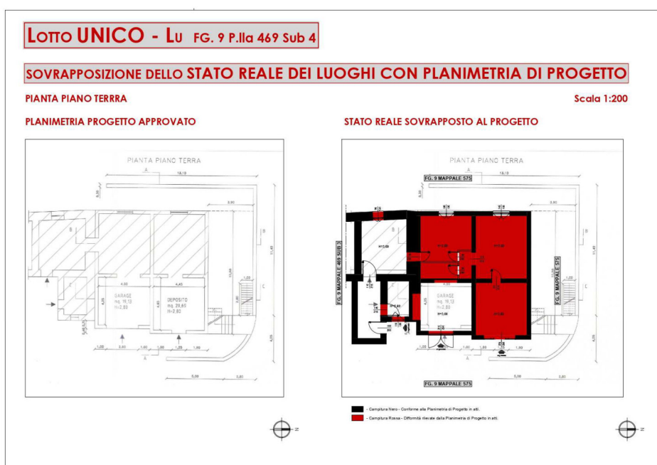
Figura 12 – Sovrapposizione Stato Reale dei Luoghi con Progetto Autorizzato Lotto Lu – PT (ALL. 10).
