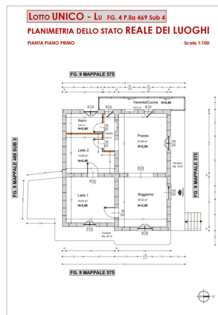
Figura 10 – Planimetria dello STATO REALE LOTTO L U – PIANO P. (ALL. 07).
