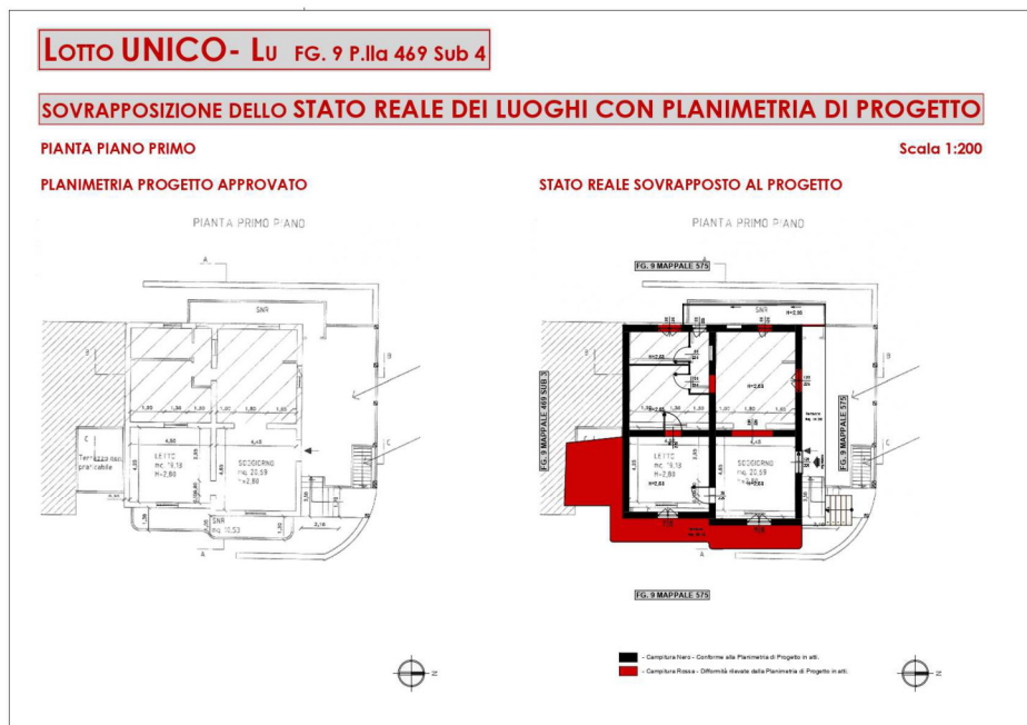
Figura 13 – Sovrapposizione Stato Reale dei Luoghi con Progetto Autorizzato Lotto Lu – P1 (ALL. 10).
