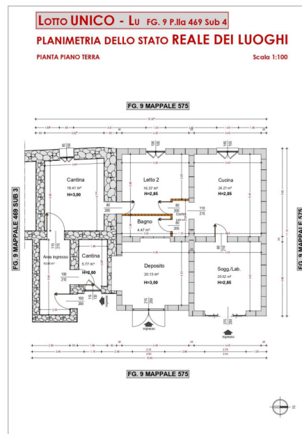
Figura 9 – Planimetria dello STATO REALE LOTTO L U – PIANO T. (ALL. 07).
