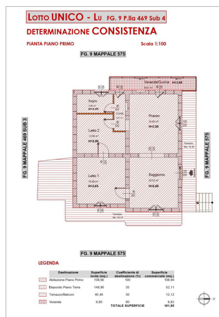
Figura 15 – Determinazione consistenza Lotto L U – PIANO PRIMO (ALL. 11).
