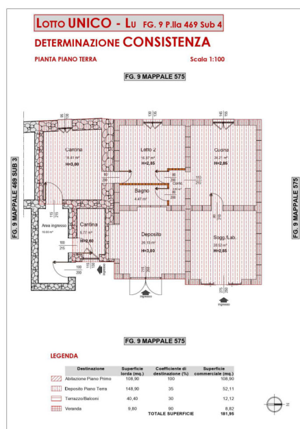
Figura 14 – Determinazione consistenza Lotto LU - PIANO TERRA (ALL. 11).
