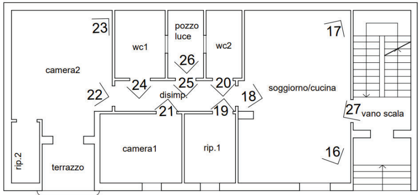
piano rialzato
