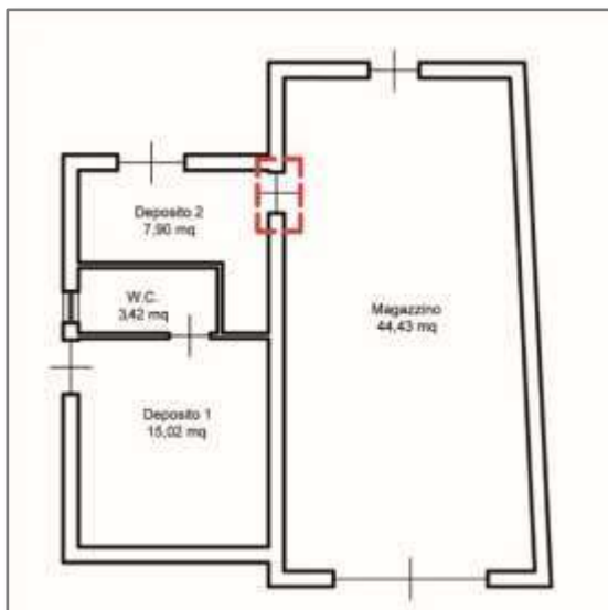
Punto c. Pianta piano terra – rilievo geometrico del 24/05/2022
