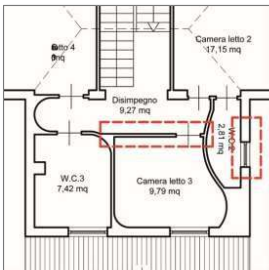
Punto b. Pianta piano primo – rilievo geometrico del 24/05/2022
