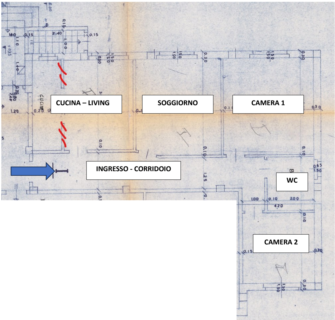
Schema ripartizione Spazi
