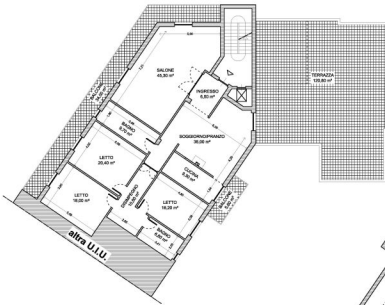
PIANTA APPARTAMENTO (foglio 12 p.la 204 sub 42)
