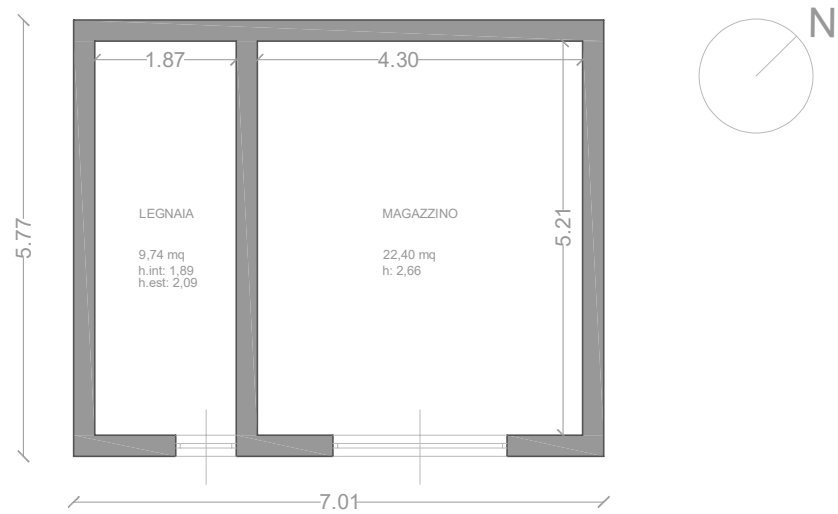
Pianta stato di fatto - scala 1:100
