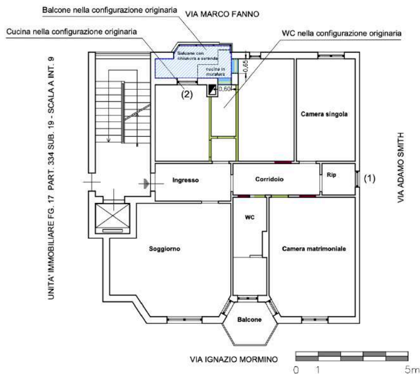
Sintesi delle difformità tra planimetria catastale in atti e stato di fatto
