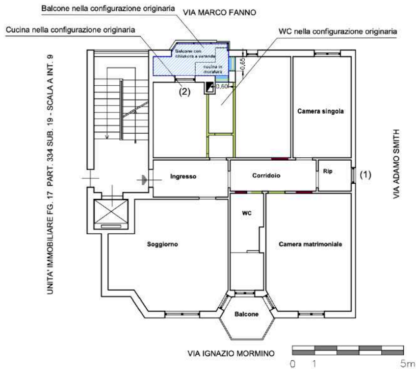
Configurazione originaria autorizzata con Licenza Edilizia n.113 del 14.03.1968
