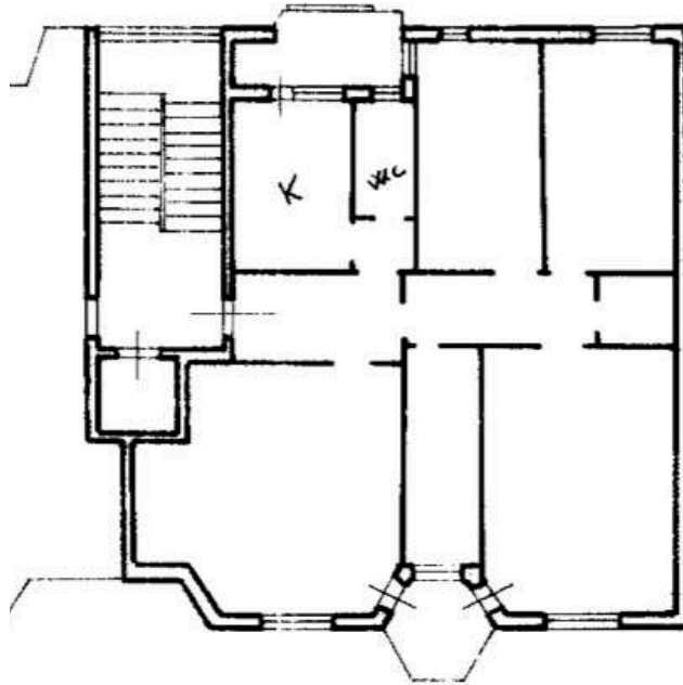
Configurazione originaria autorizzata con Licenza Edilizia n.113 del 14.03.1968
