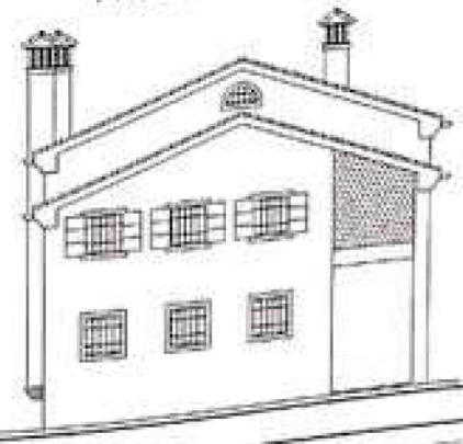
PROSPETTO NORD
