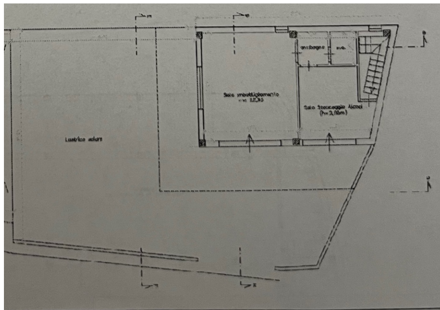
Elaborato grafico Permesso di costruire n. 14/22
