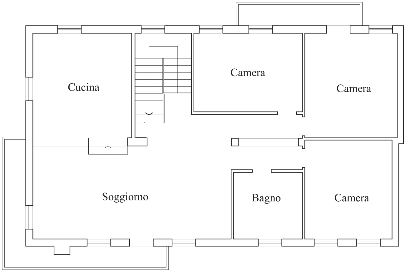
PIANO PRIMO - 1:100
