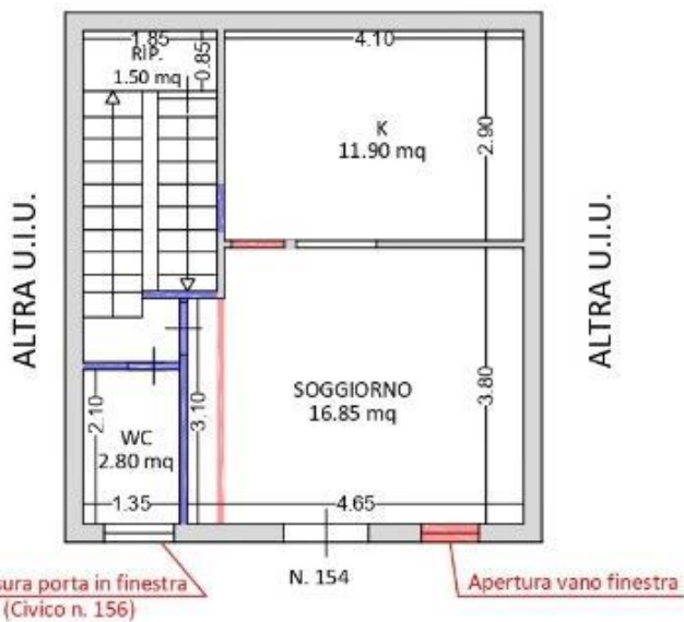
VIA ANTONIO GRAMSCI PIANO TERRA H=3.00 m
