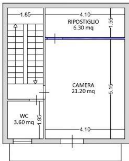
PIANO SECONDO H=3.00 m
