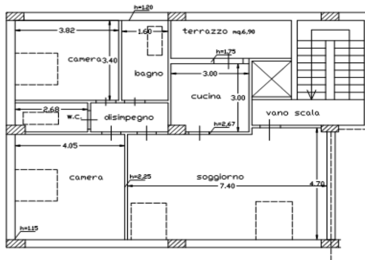
PIANTA PIANO QUARTO mansardato fg. 127 part. 321 sub 45
