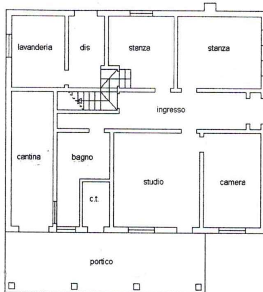
PIANO PRIMO H=2.80
