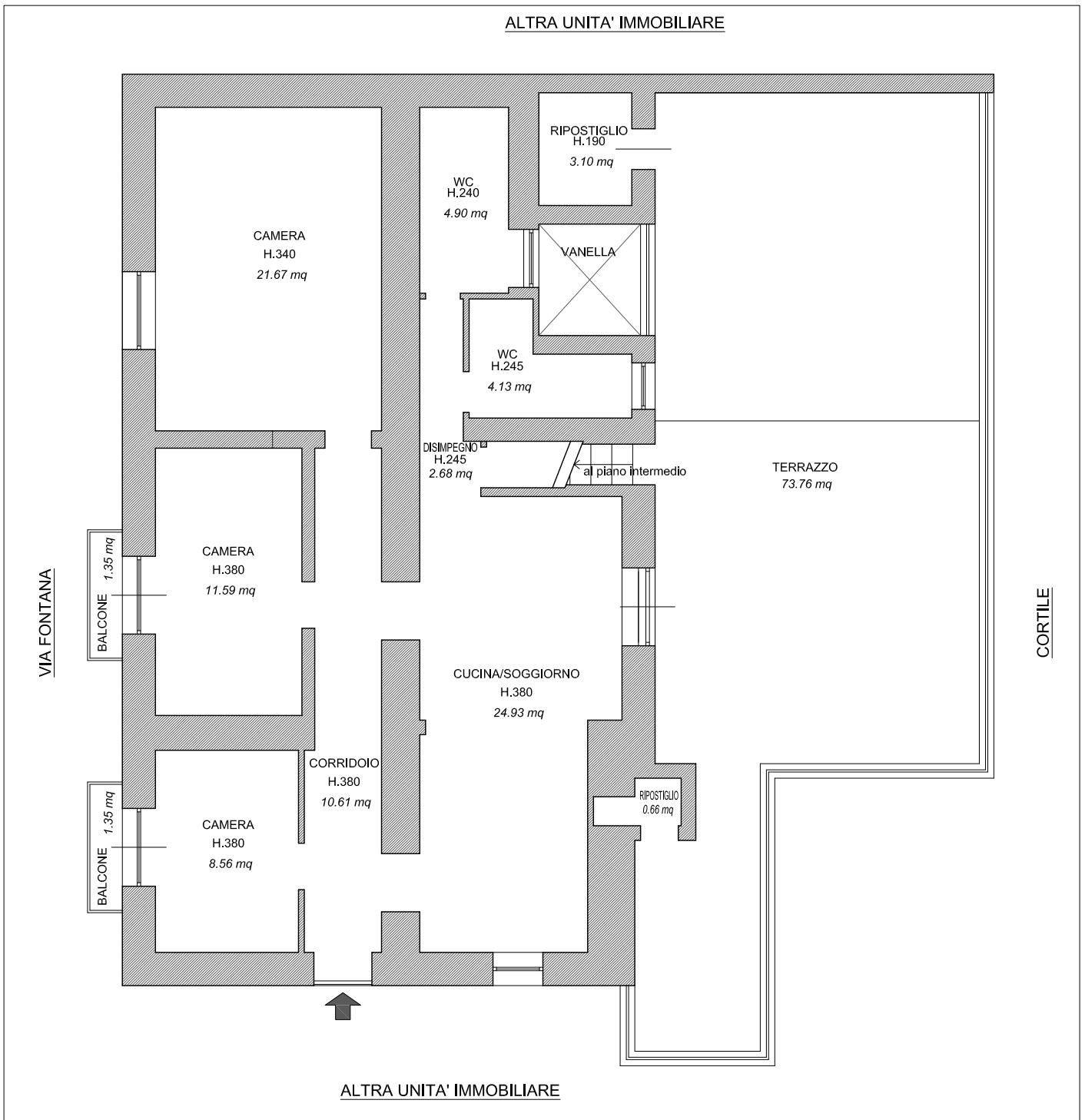
PIANTA PIANO 2°
