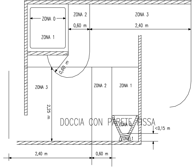
VARIANTE CON VANO SOTTOVASCA
