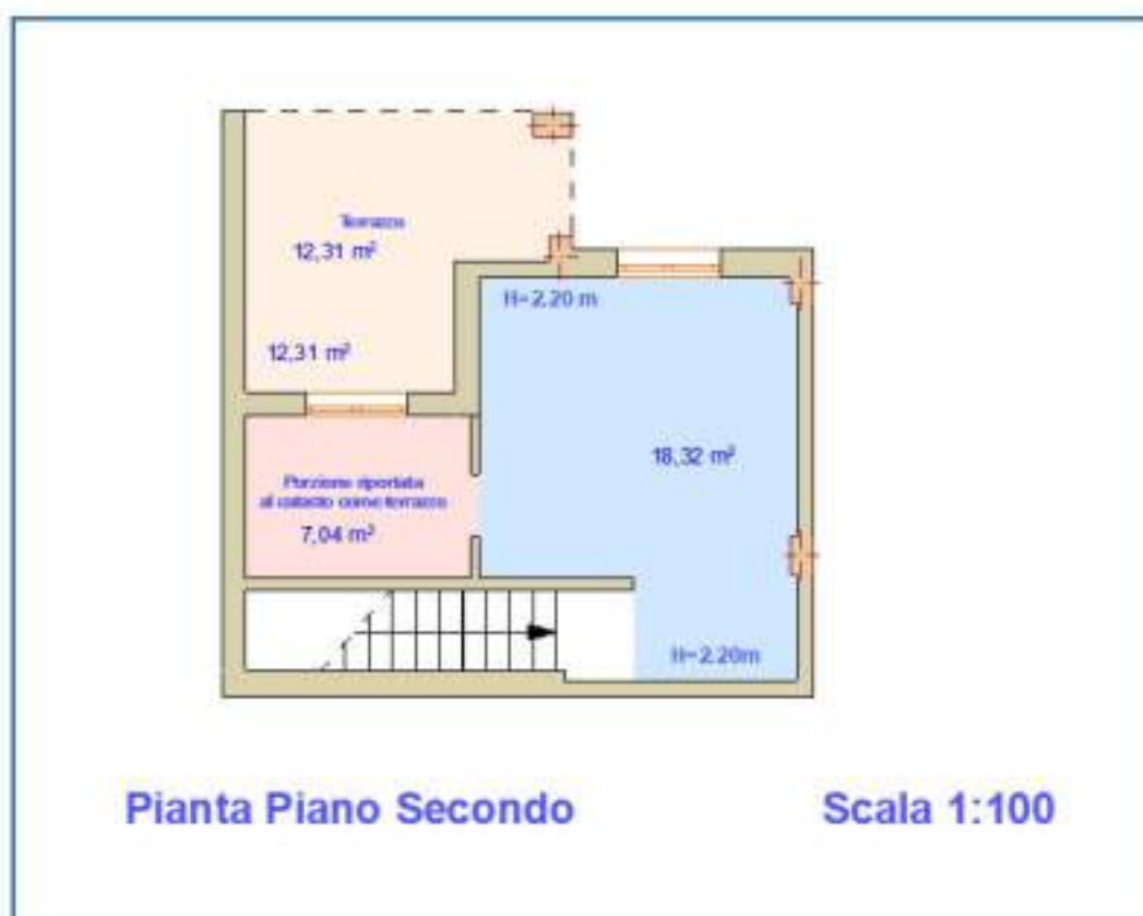
Figura 2: Planimetria di rilievo piano secondo.
