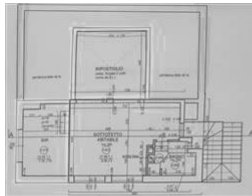
Planimetria sottotetto come da PE 33/07
