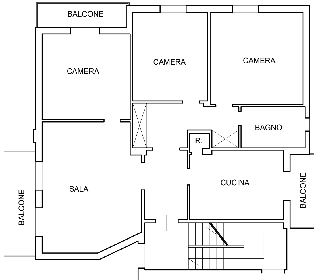
PIANO PRIMO H = 2.80
