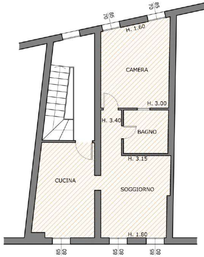
Figura 3. Planimetria immobile.
