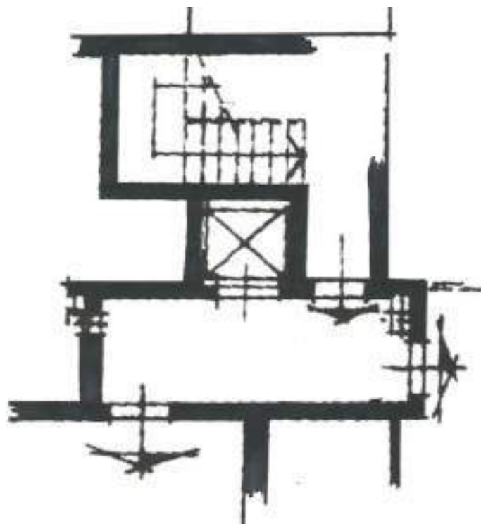
PIANTA PIANEROTTOLO
