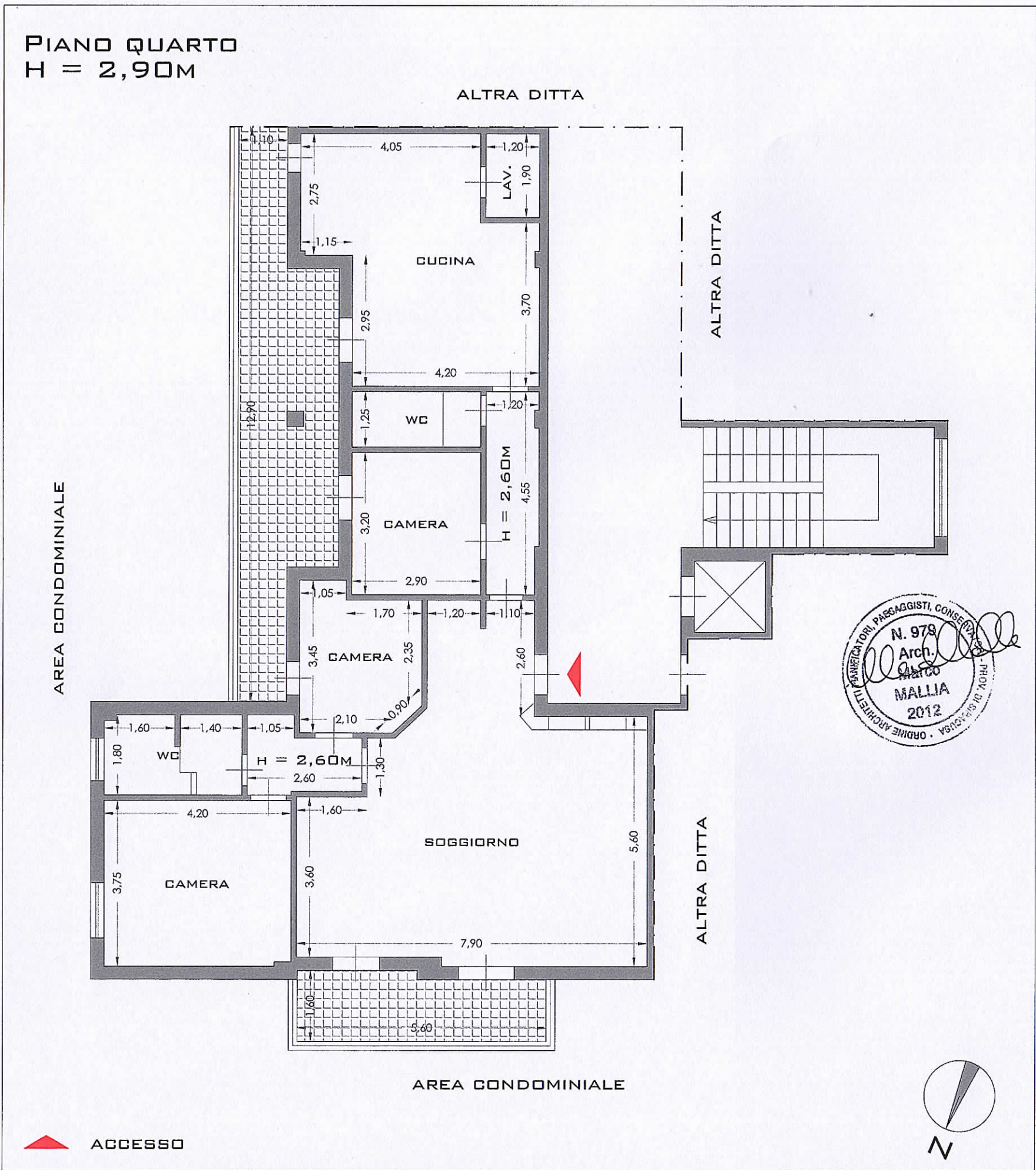
PLANIMETRIA DEGLI IMMOBILI_STATO DI FATTO_1:100 LOTTO DI VENDITA N.2
