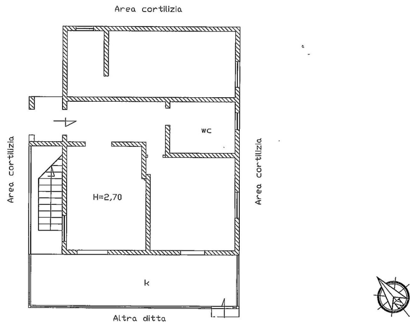
Fig.3 - Pianta piano terra
