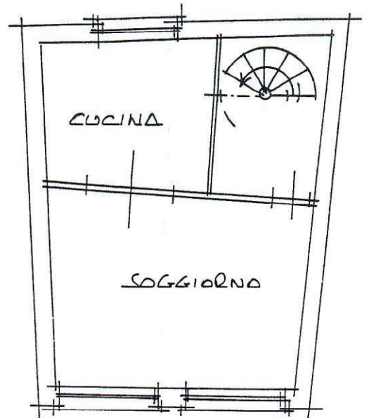
PIANO TERZO H. 2.88
