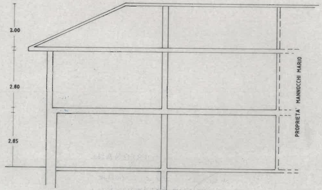
SEZIONE A-B
