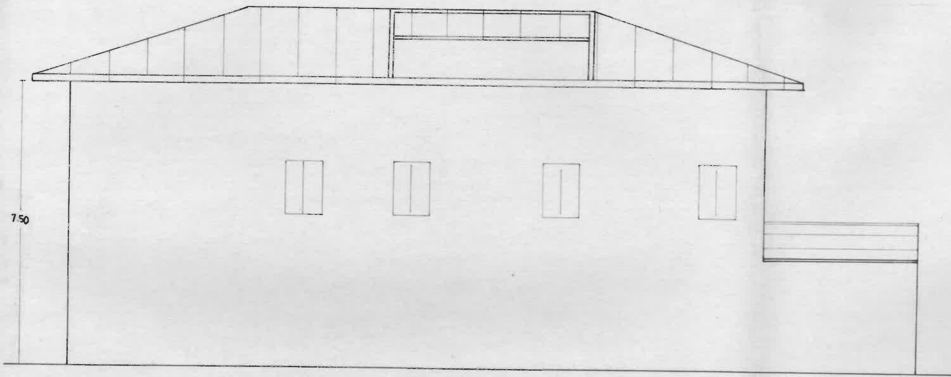
PROSPETTO NORD
