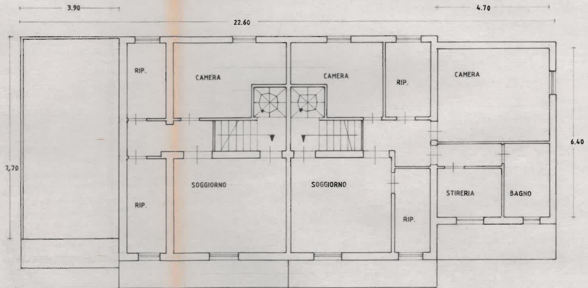
1° PIANO
