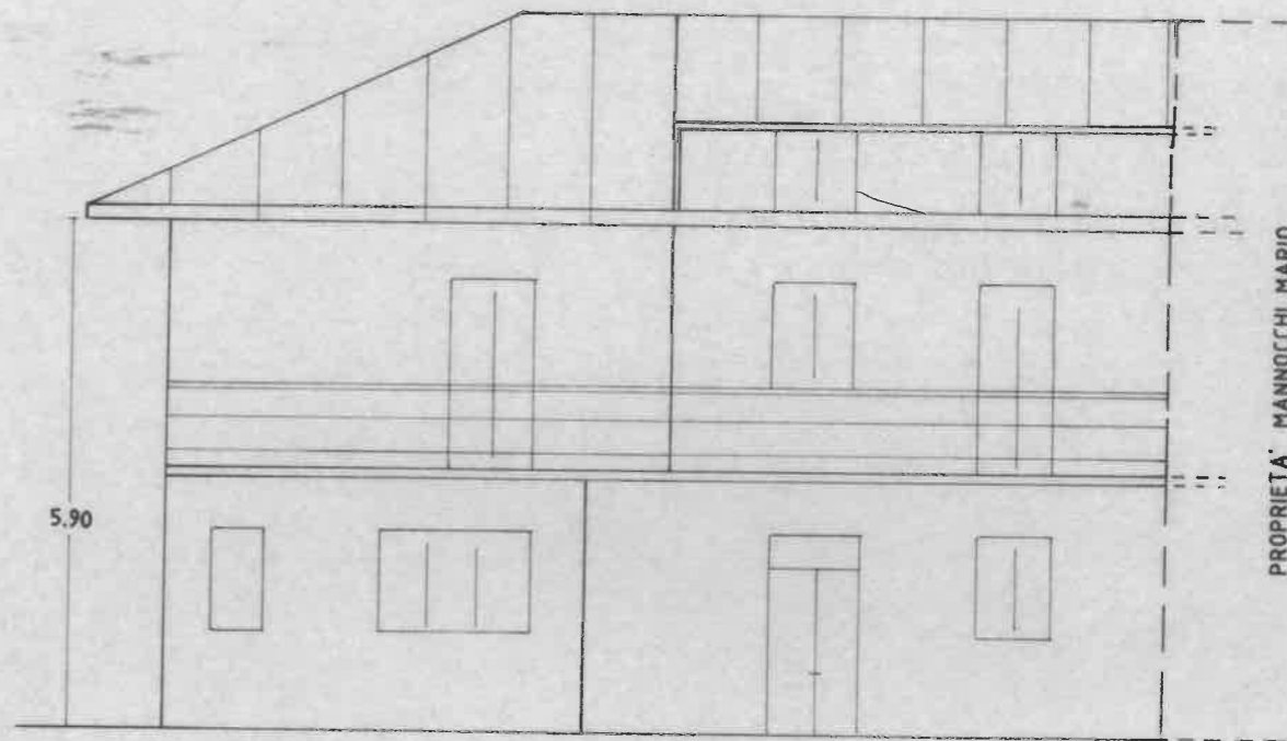
PROSPETTO SUD
