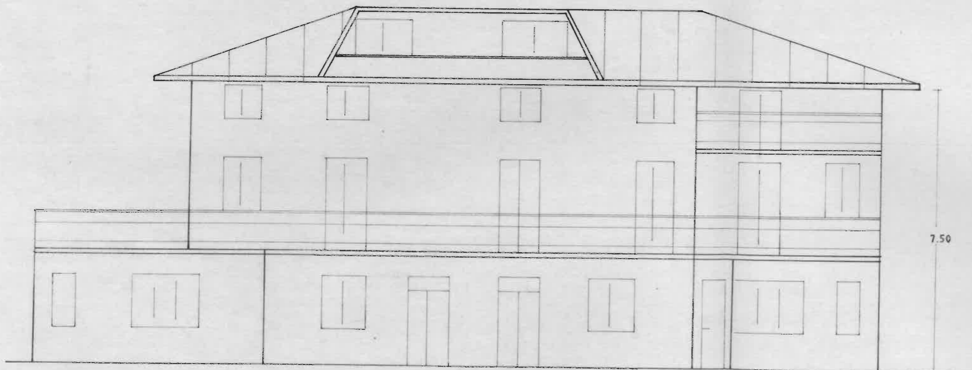
PROSPETTO SUD
