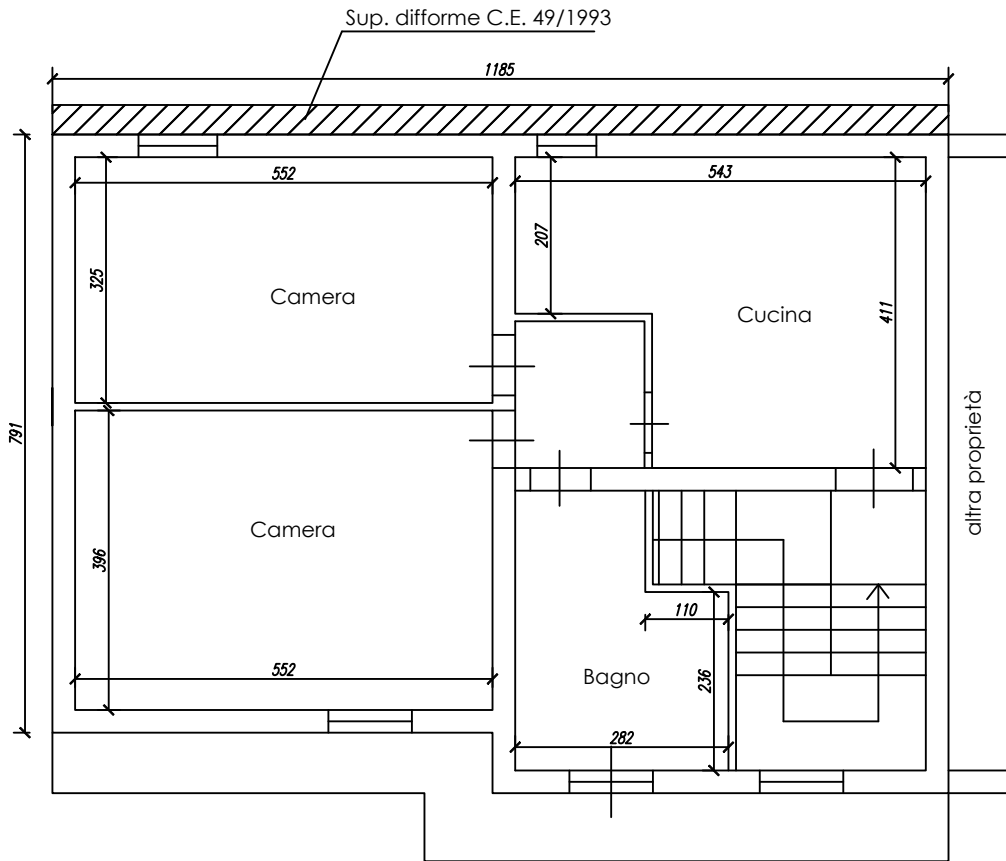
PIANO PRIMO
