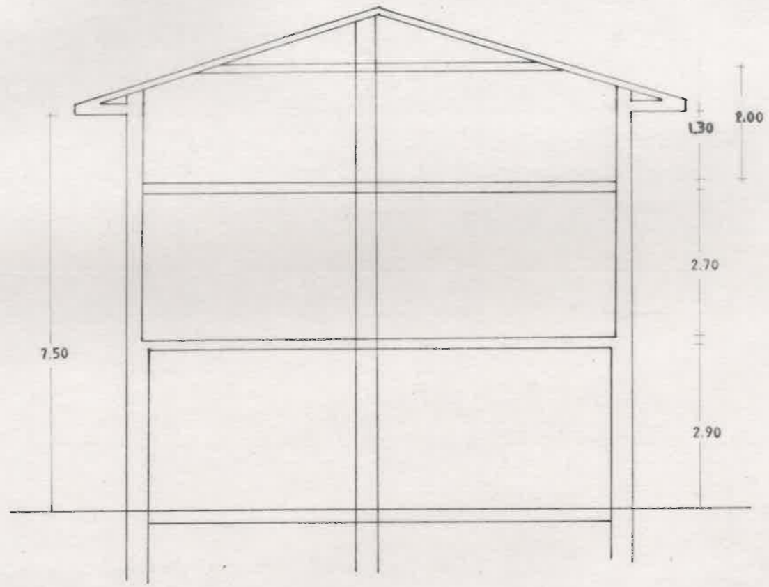
SEZIONE
