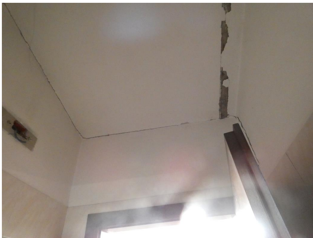
Presenza fotografica 57 – Vista Interna Antibagno: Dettaglio presenza di stato fessurativo sull' intradosso del solaio Piano Primo
