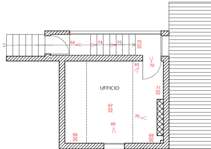
PIANTA PIANO PRIMO scala 1:100
