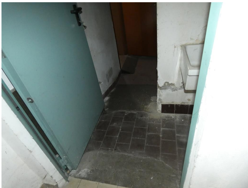
Presafotografica 13 – Vista Interna: Ingresso al vano del sottoscala (Porta REI), con dettaglio dello scrostamento dell’intonaco viziato dalla presenza della risalita capillare dell’umidità dal terreno
