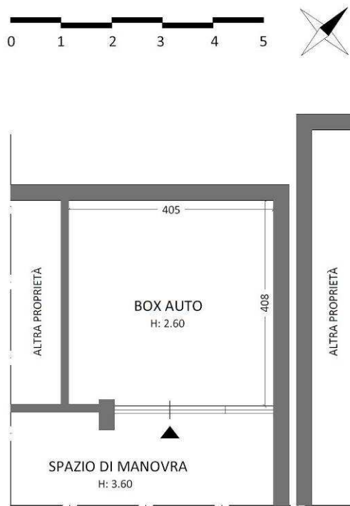
Pianta Piano Seminterrato Scala A
