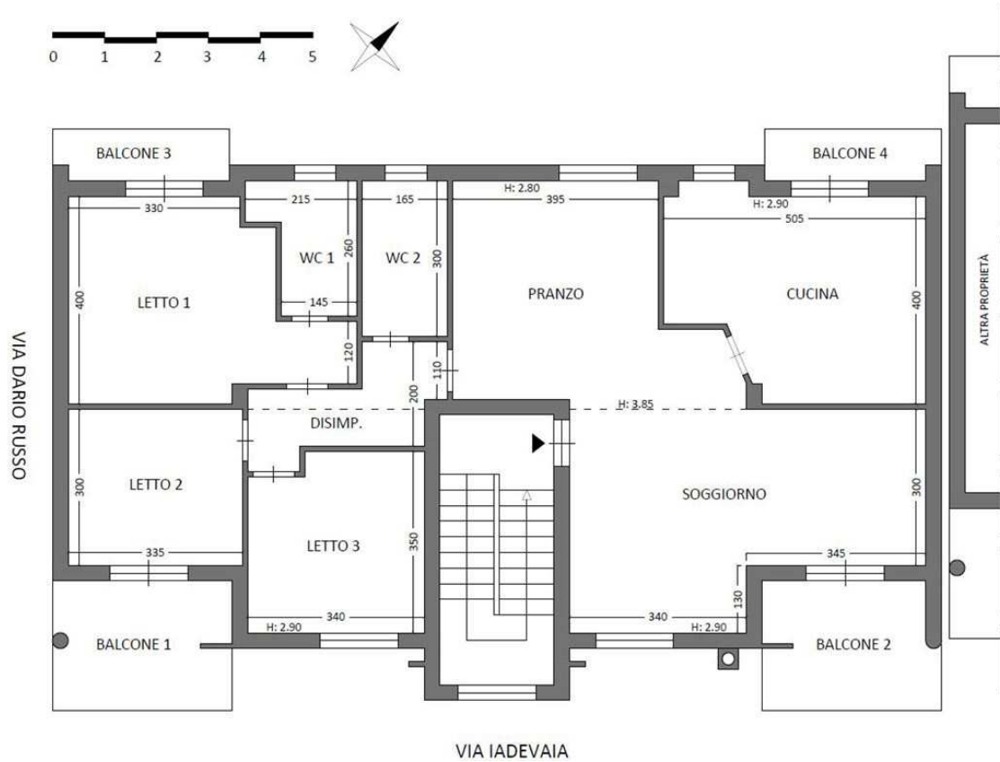
Pianta Piano Secondo Scala A Interno 5
