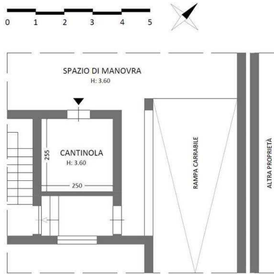
Pianta Piano Seminterrato Scala A
