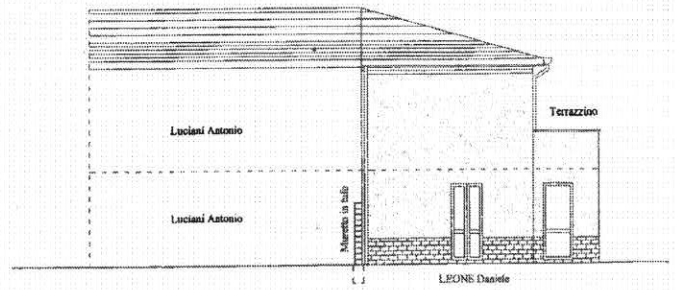
PROSPETTO POSTERIORE
