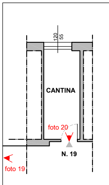
PIANTA STATO DI FATTO CANTINA Via Cartagine,15 - Piano 8° Int. 18
