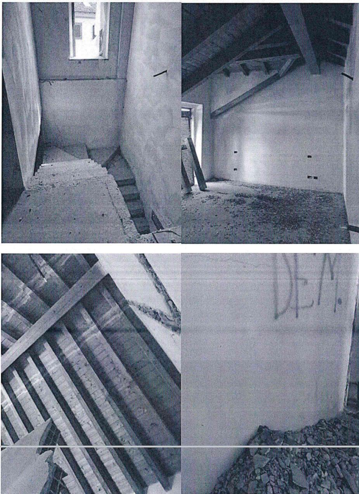
Piano terra e primo sub. 121 A - stato attuale finiture
