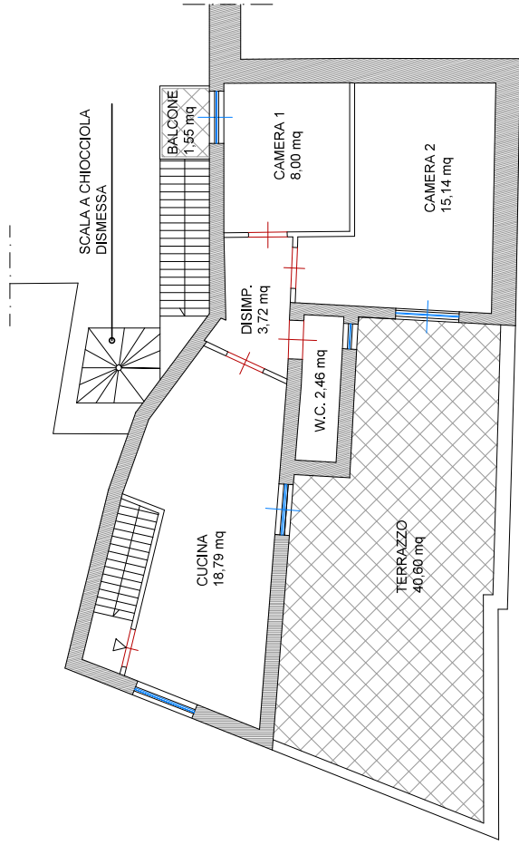
PIANO SECONDO
